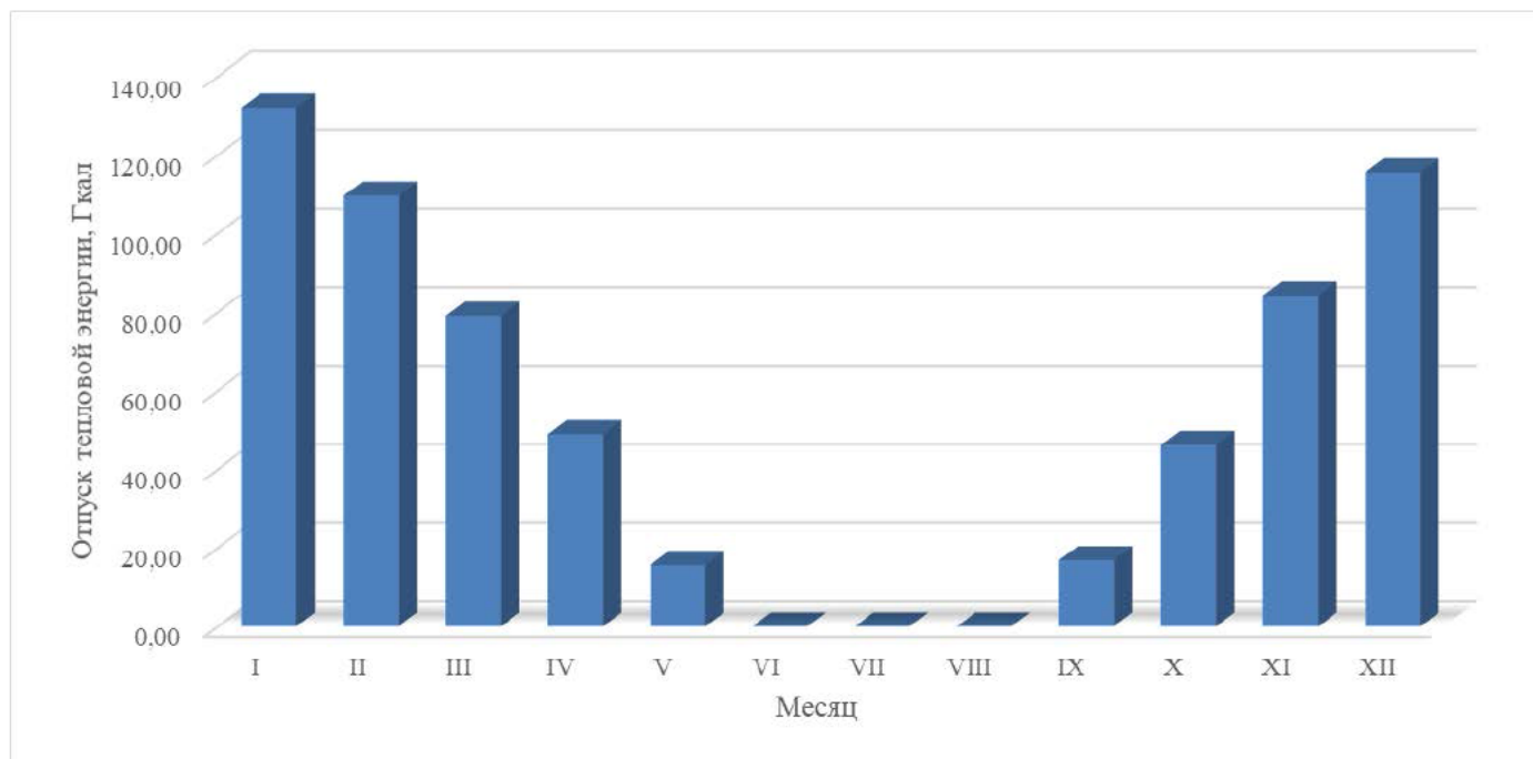
Рисунок 1.3 – Оптимальный температурный график отпуски тепловой энергии для котельной с. Лукашкин Яр
